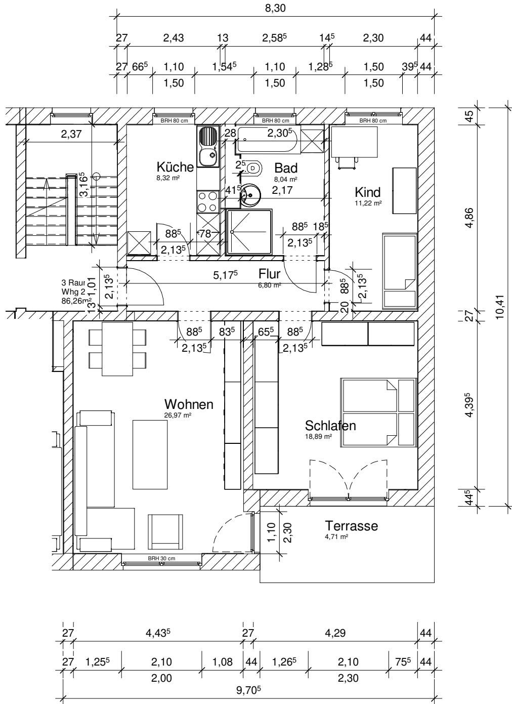
Erdgeschoss Wohnung 2
